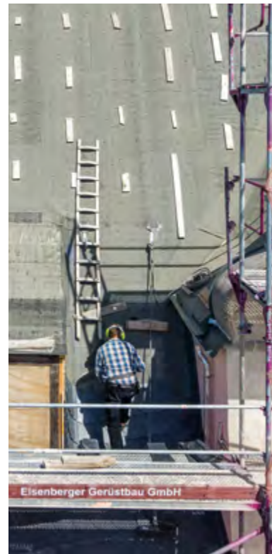
Schieferarbeiten in Altdeutscher Deckung
