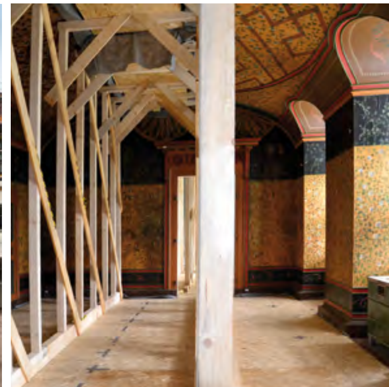
Deckenabstützungen zum Schutz historischer Räume unter dem Dachgeschoss
