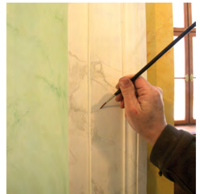
Gotha, Schloss Friedenstein, Wiederherstellung der Marmorierung im Herzoglichen Treppenhaus
