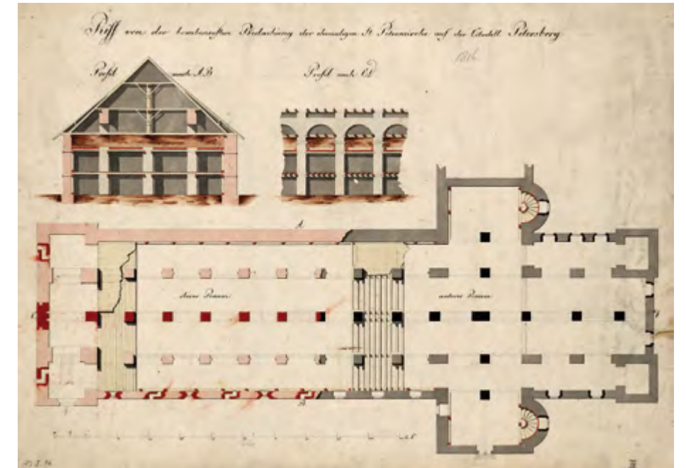
Nicht vollständig realisierte Planzeichnung für den Umbau der Kirche zum Proviantmagazin, 1818
