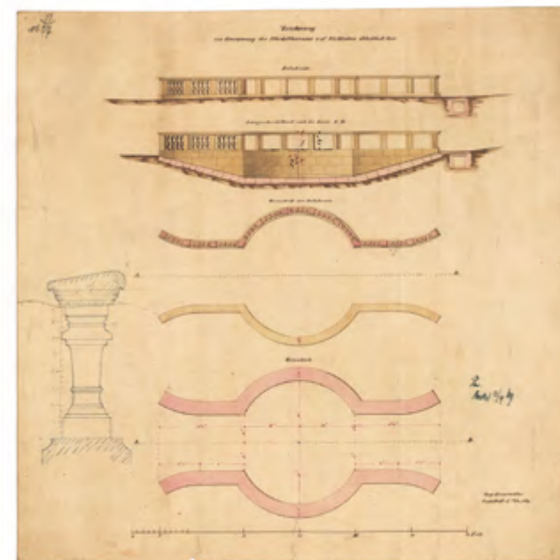
August Bauermeister, Plan der Pferdeschwemme, 1869
